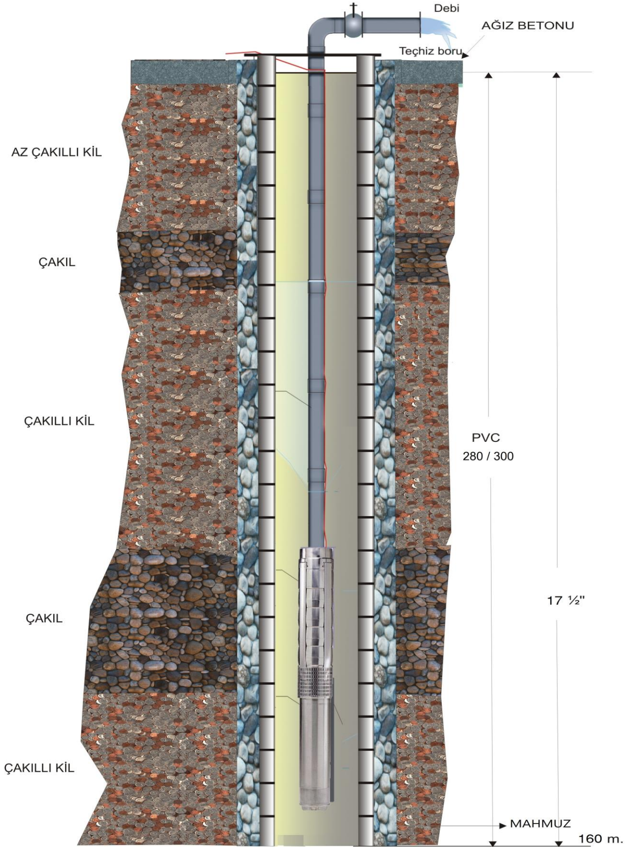
EK -1 ADET SONDAJ KUYU KESİTİ
