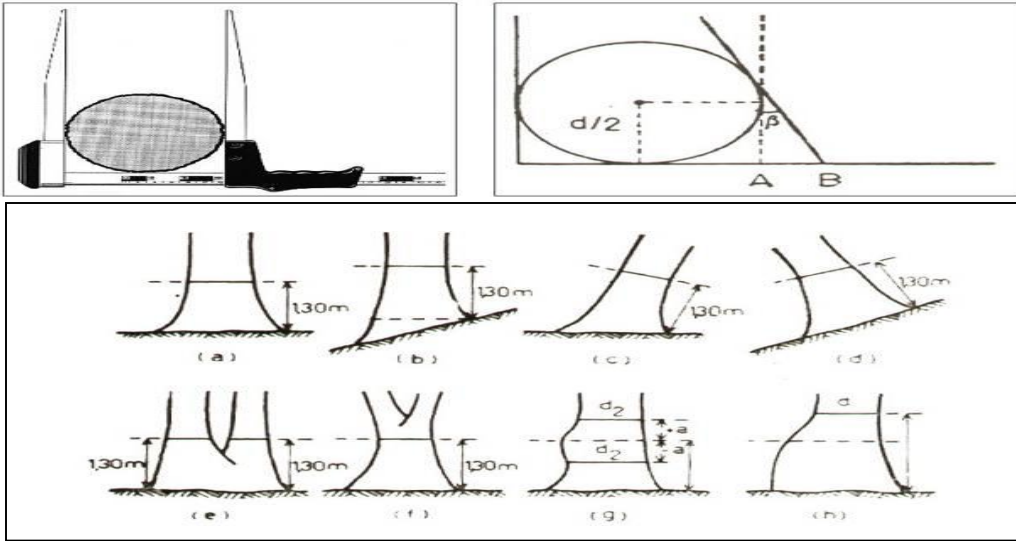
Şekil 12. Çap Ölçerinin Kullanım Şekli
