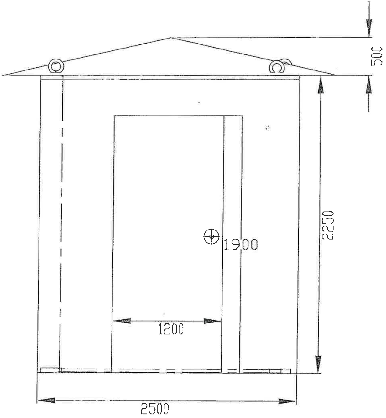
ÖN GÖRÜNÜŞ
